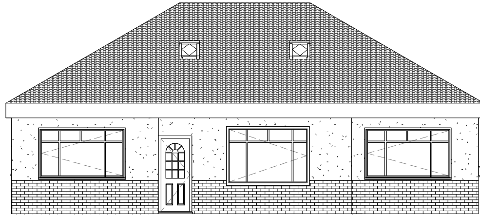
1 North 1 : 100
