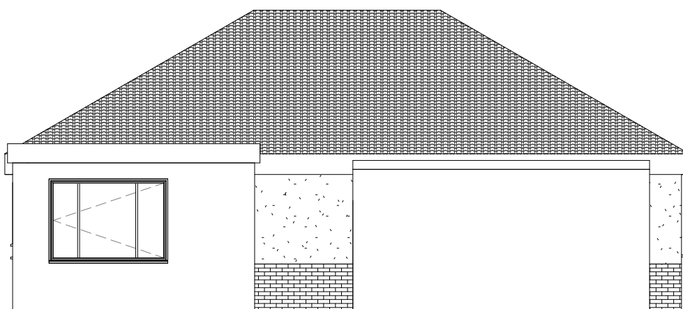
3 South 1 : 100
