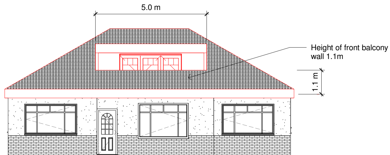
1 North 1 : 100
