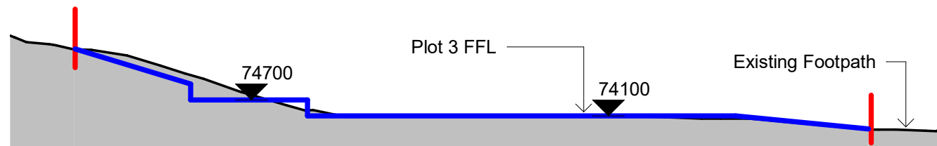
3 Section 3 1 : 200
