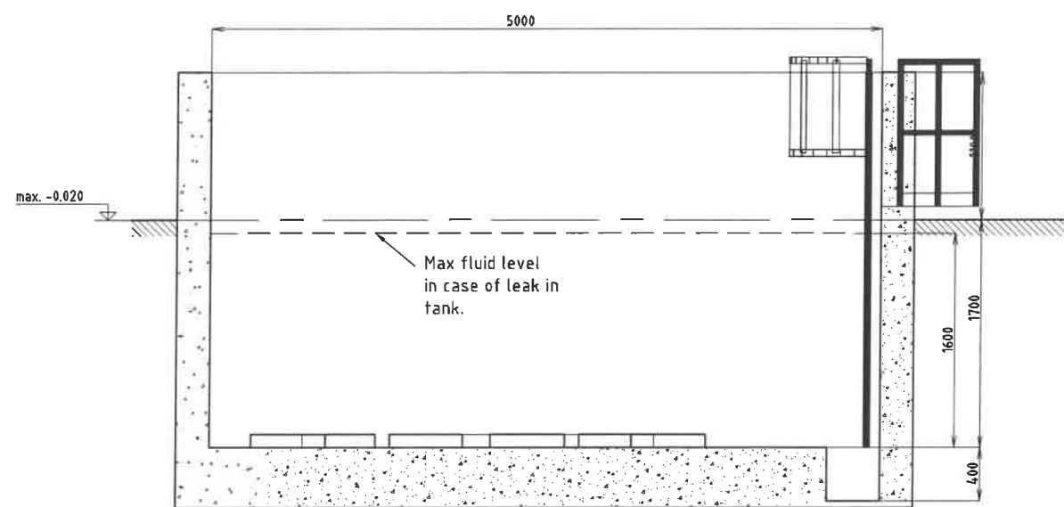
View A-A
