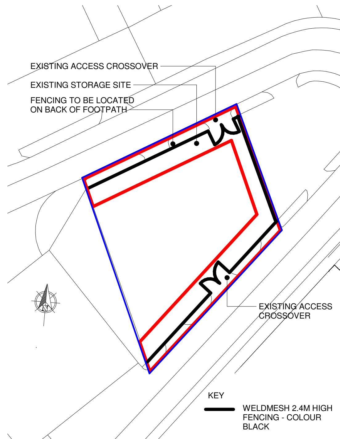
BLOCK PLAN 1 : 500
