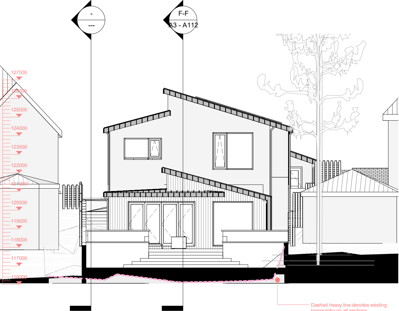
SECTION B-B 1 : 125
