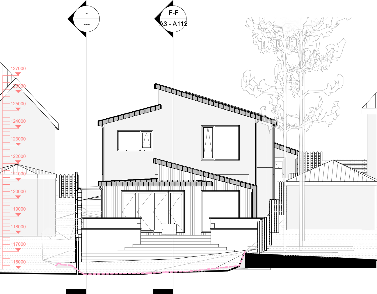
SECTION A-A 1 : 125
