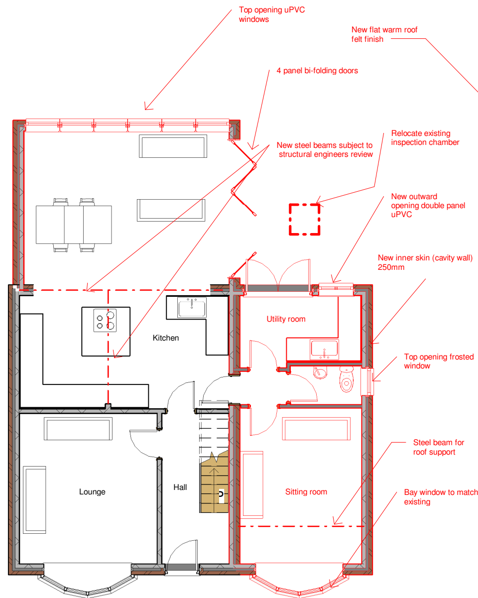
1 GF 1 : 100
