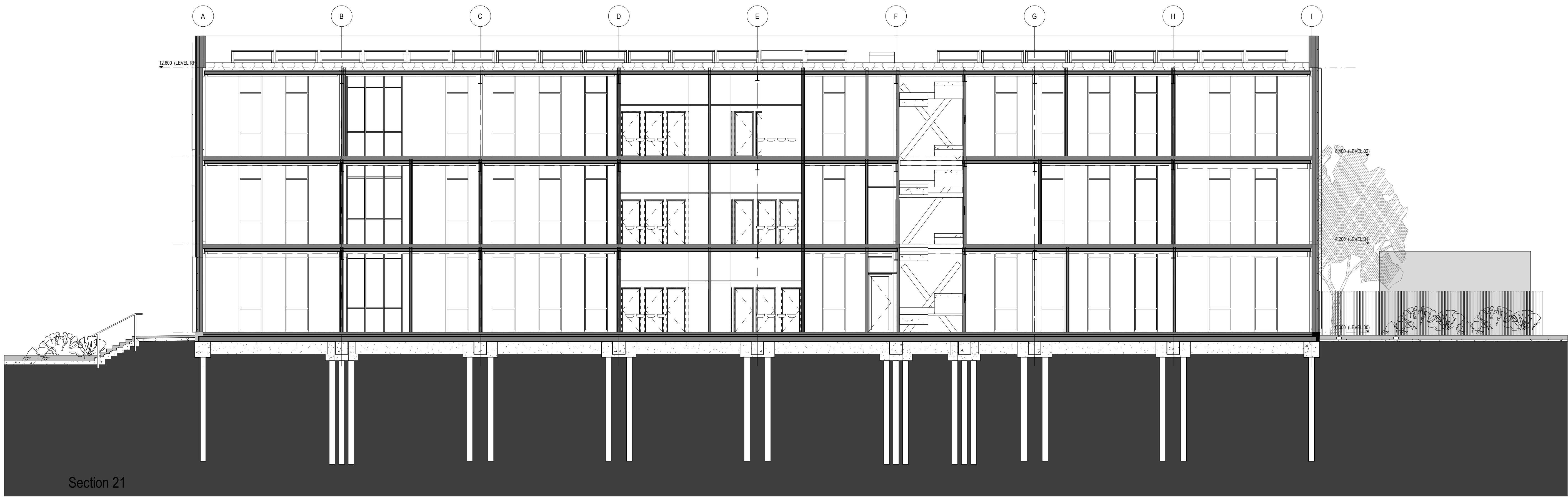
Section 21 1 : 100
