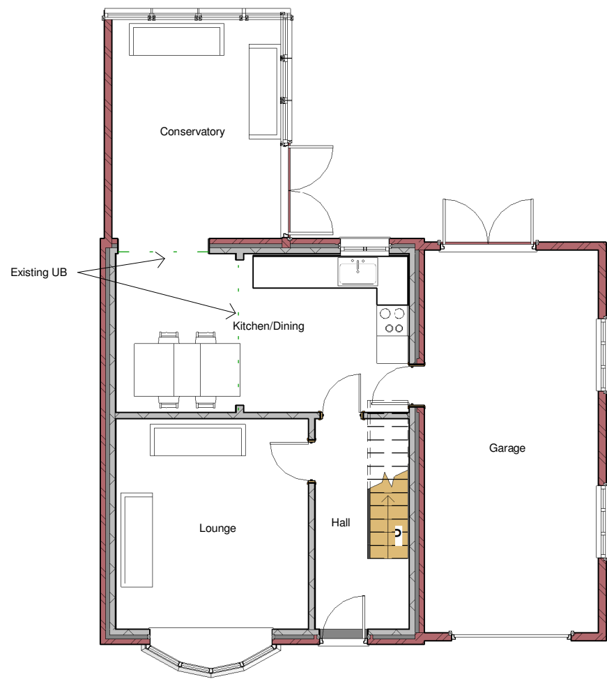
1 GF 1 : 100
