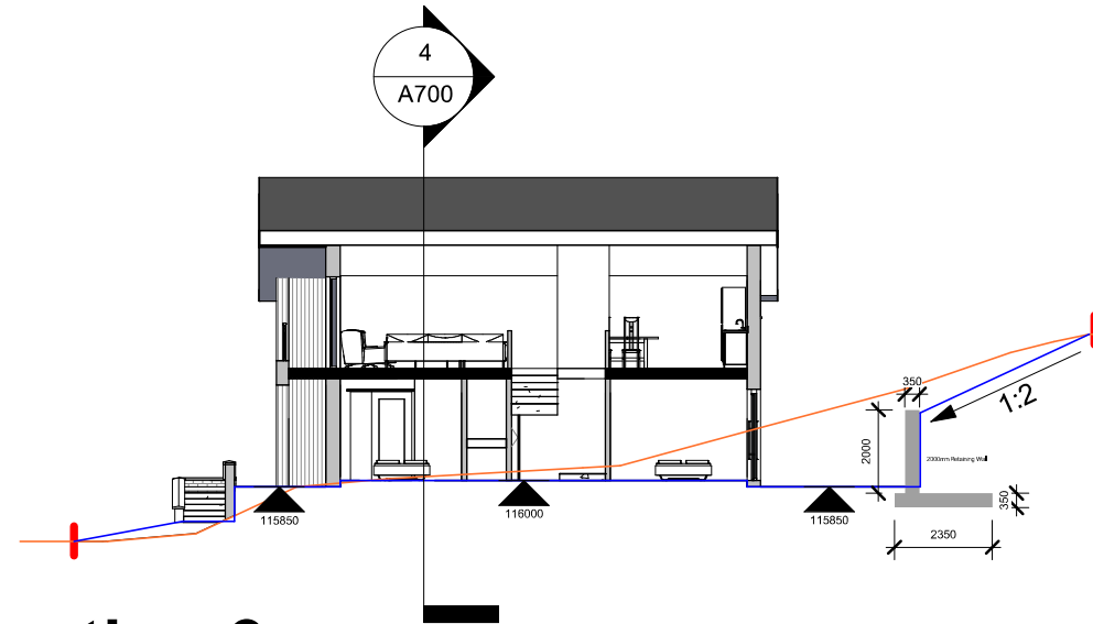
3 Section 3 1 : 200
