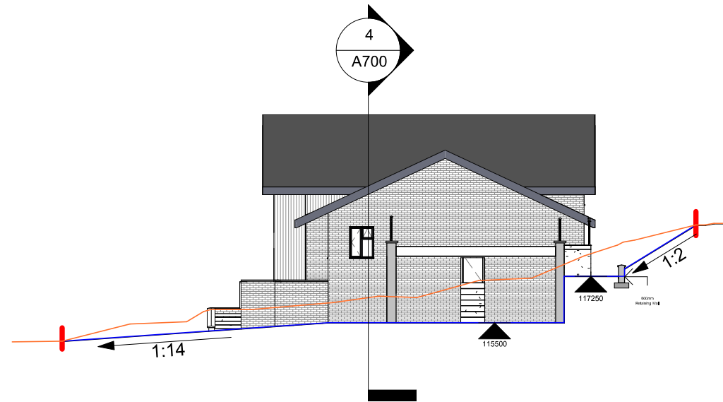
1 Section 1 1 : 200
