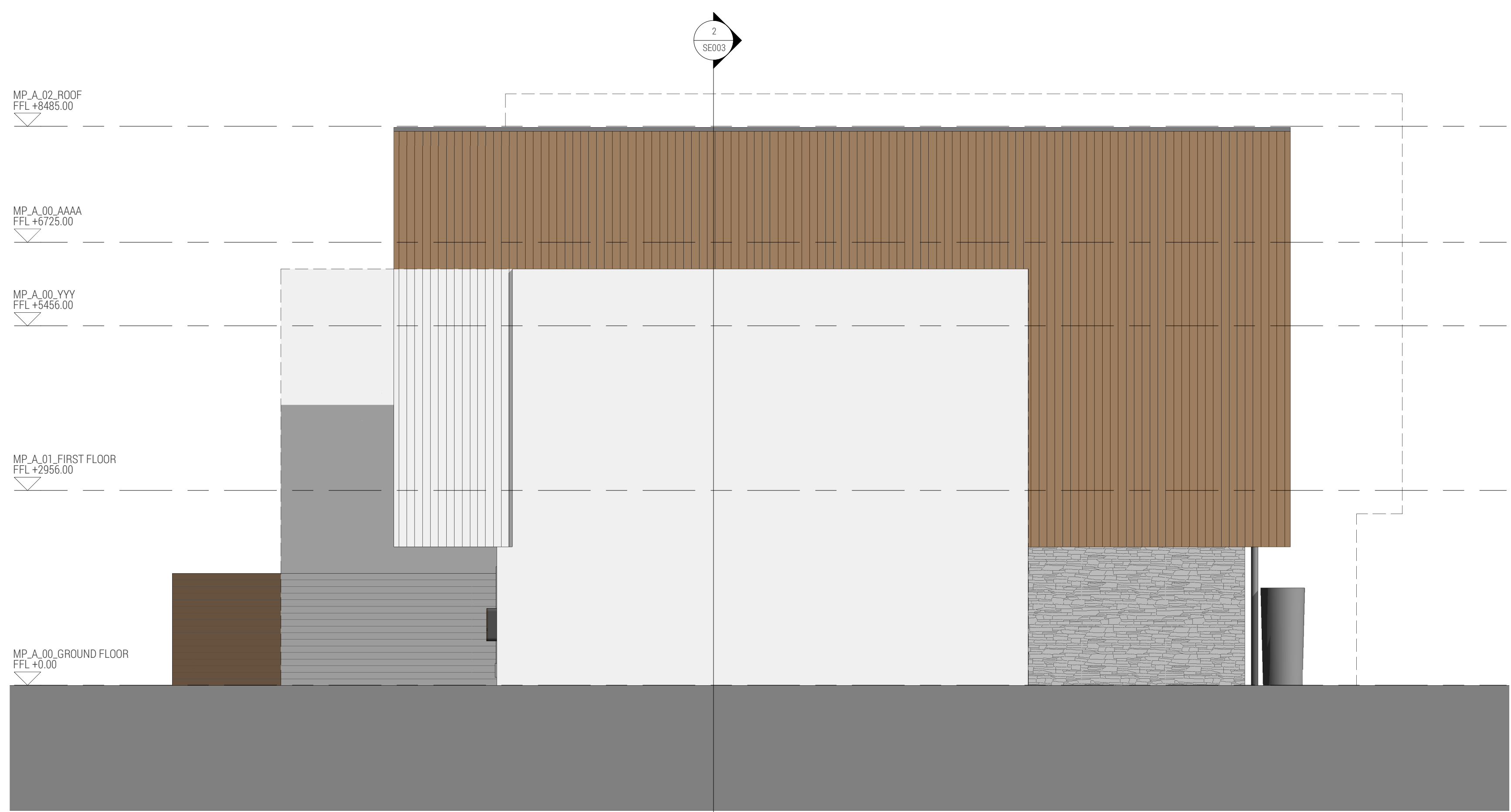
2 | Elevation 02
