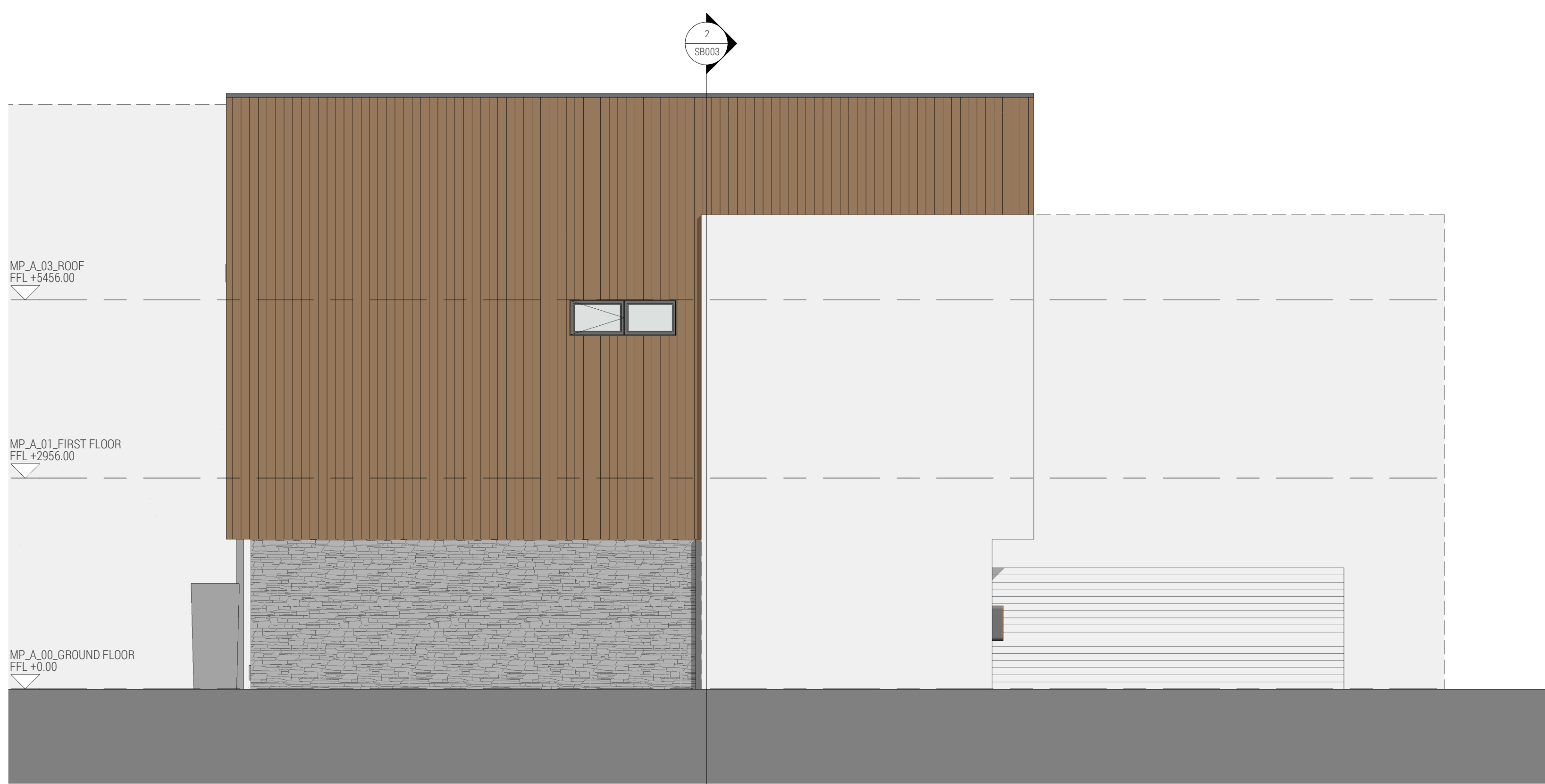
4 | Elevation 04
