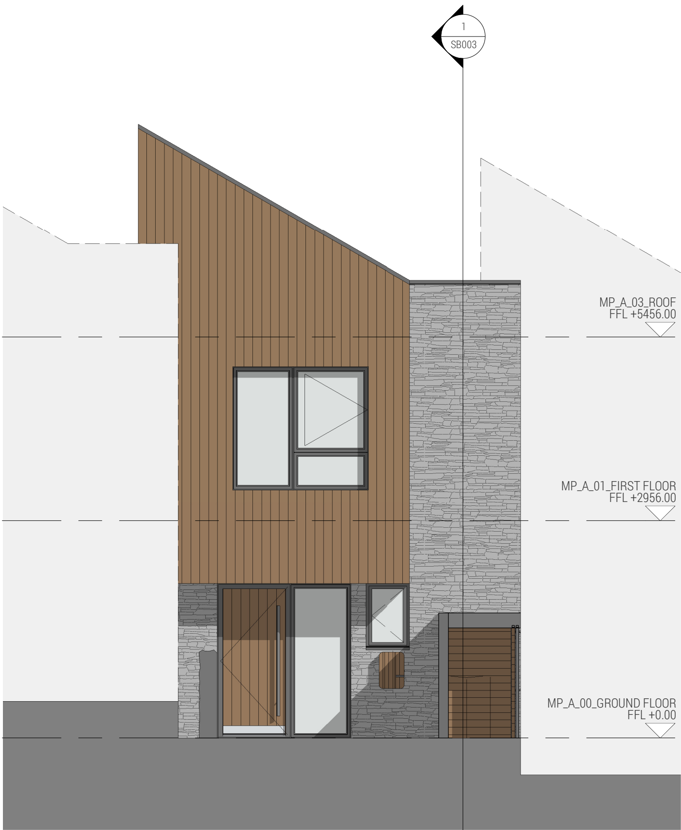
1 | Elevation 01
