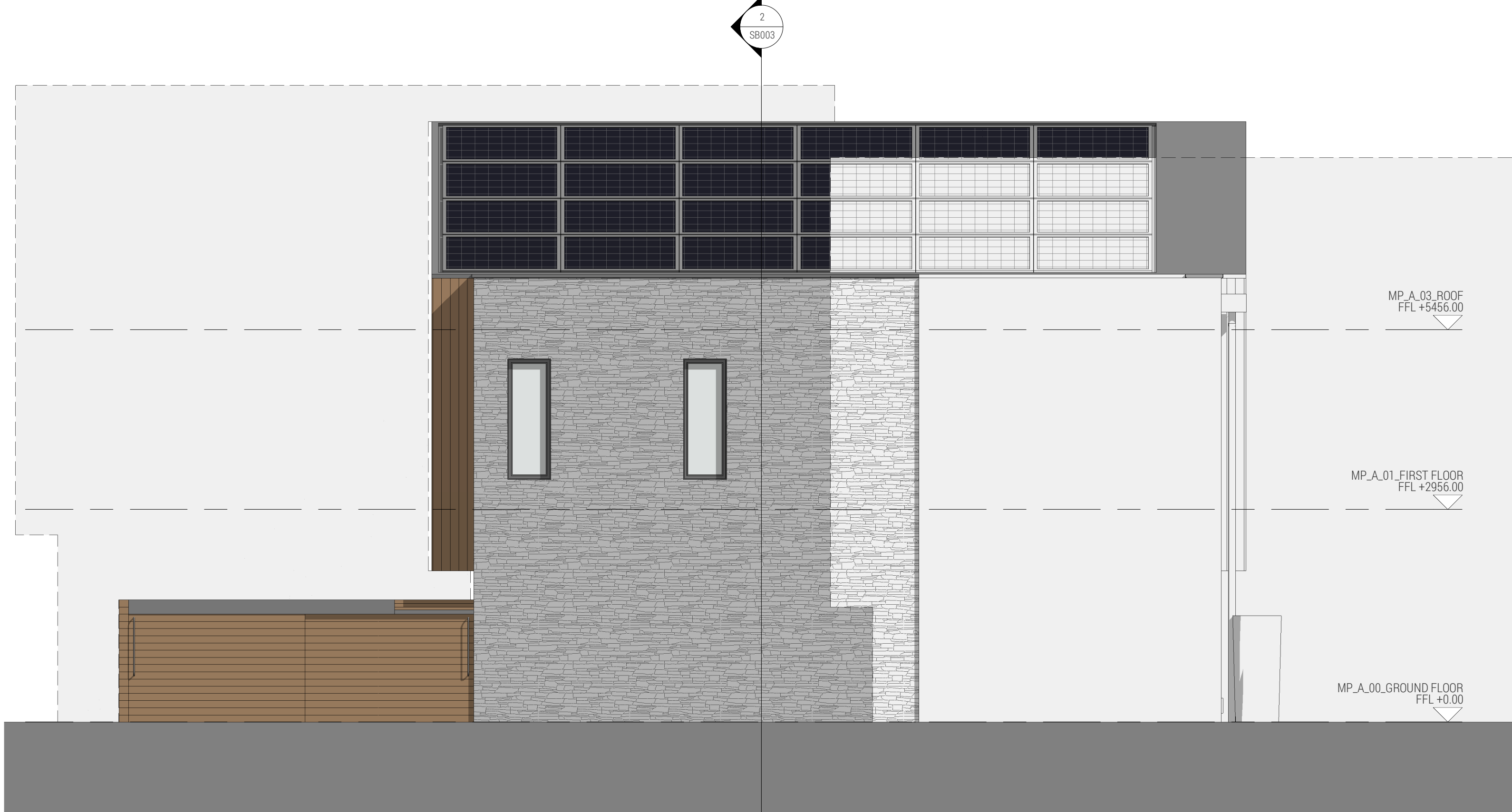
2 | Elevation 02
