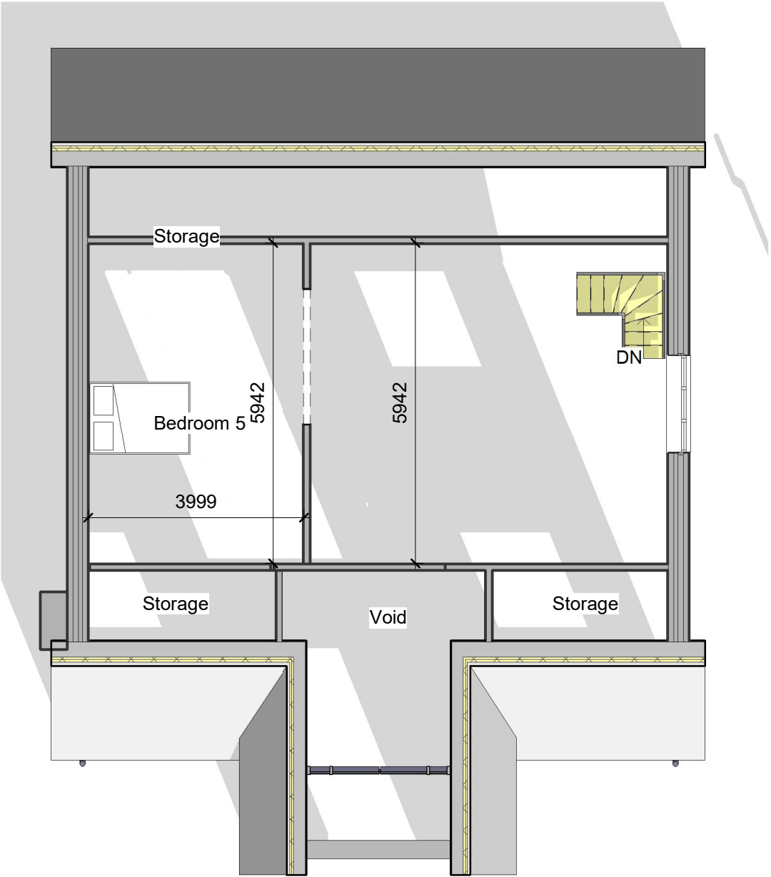
1 SF Plan 1 : 100
