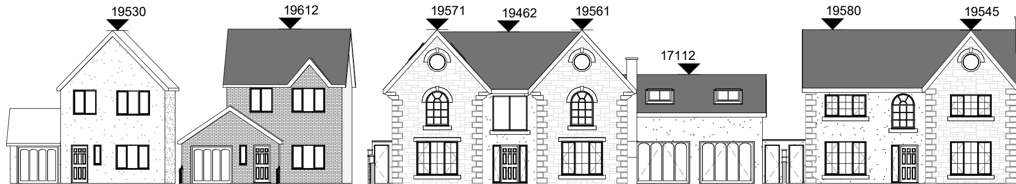
1 Front 1 : 200
