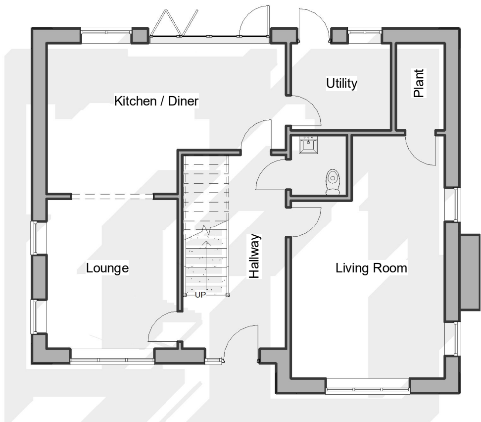
1 Level 0 - House 2 1 : 100
