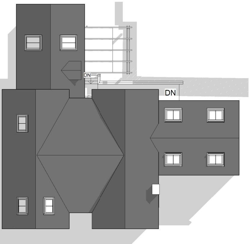
4 Roof Plan 1 : 200
