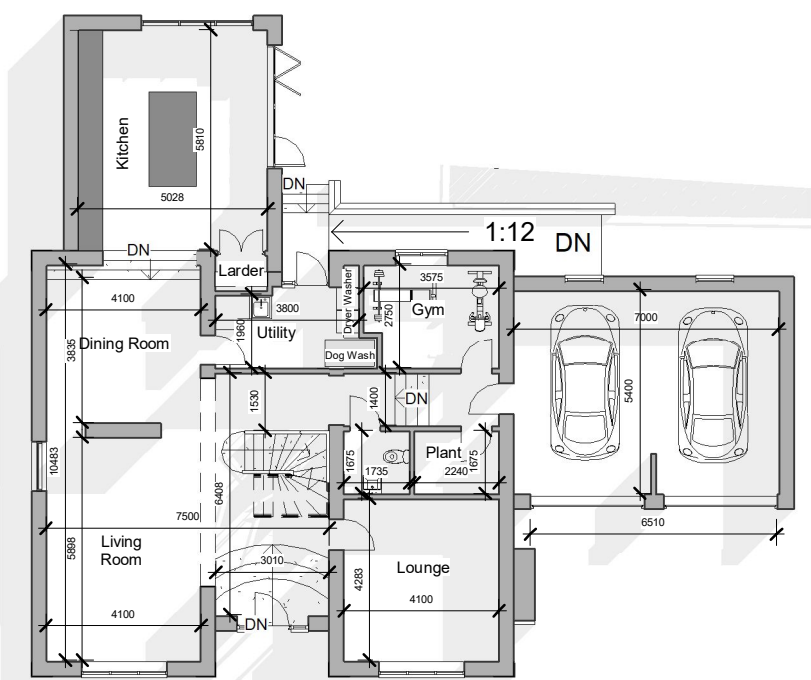
1 Level 0 1 : 200
