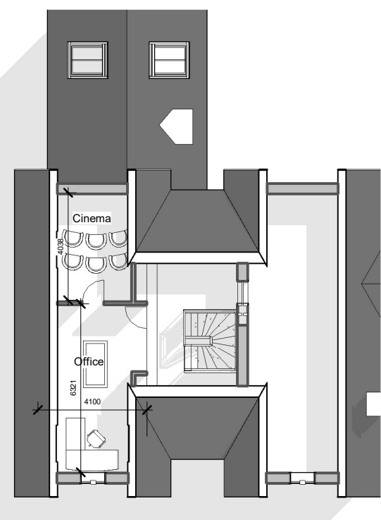
3 Level 2 1 : 200
